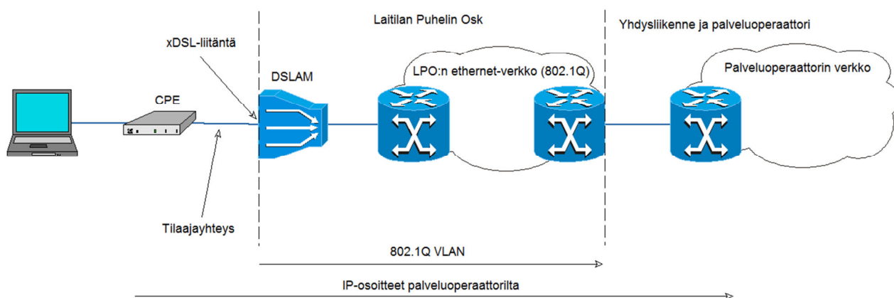
Kuva 1. Ethernetillä toteutettu yhdysliikenne
